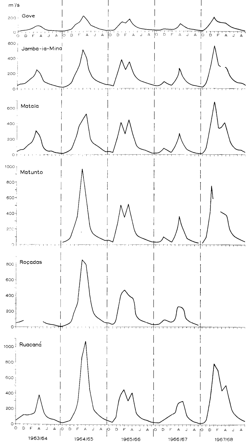
Fig. 2 — Caudais médios mensais do Cunene (em metros cúbicos por segundo).
