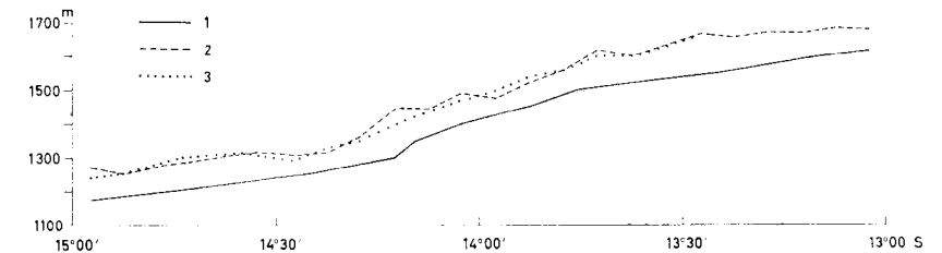
Fig. 7 — Declives do rio e da aplanção entre as latitudes 13^{\circ} 00' e 15^{\circ} 00' . 1 — Perfil longitudinal do rio; 2 — declive da aplanção obtido por estatística de cotas de duas faixas paralelas ao rio (fig. 9); 3 — declive da mesma aplanção obtido por estatística de cotas de uma faixa com 30' de largura (fig. 8).
