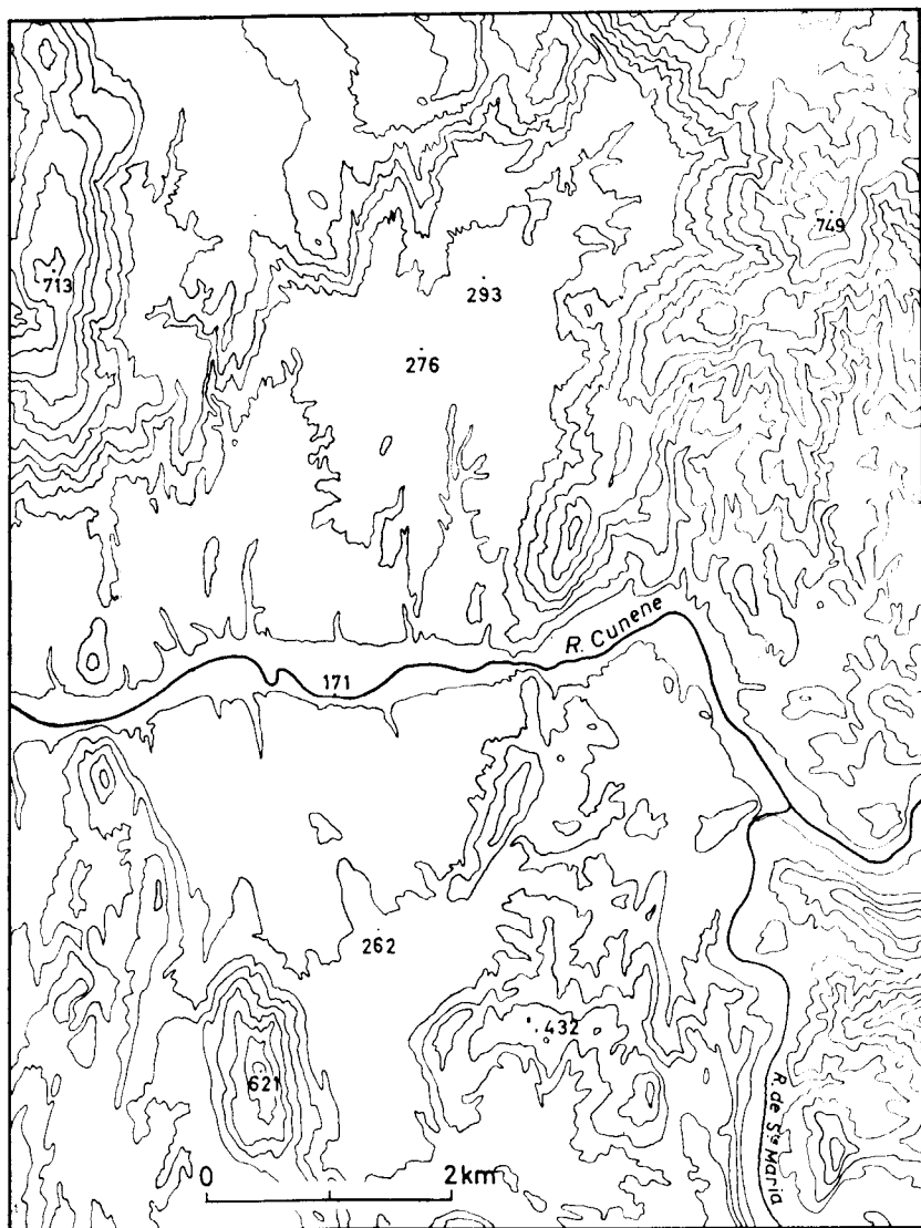
Fig. 14 — A depressão de Ongomulé. Curvas de nível equidistantes de 50 m.
