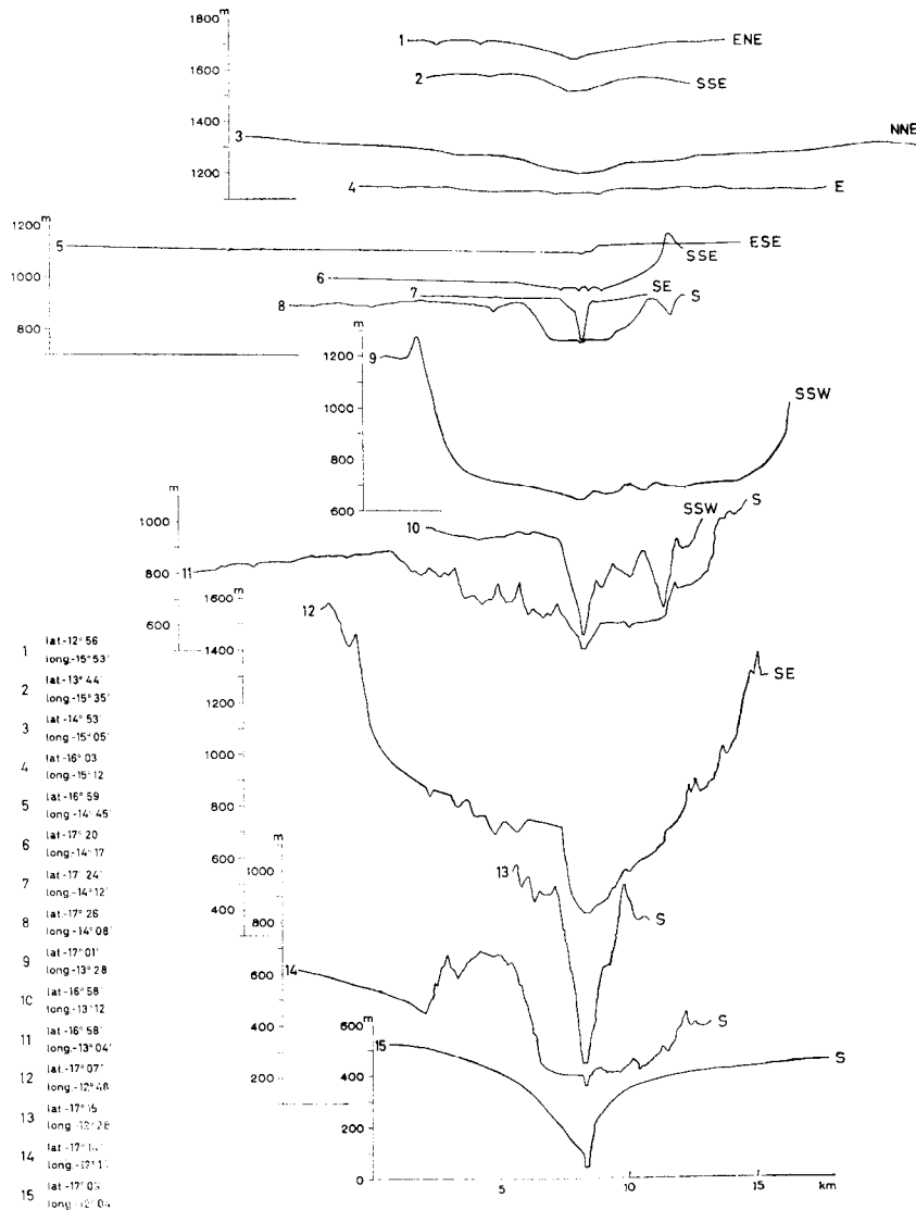
Fig. 4 — Perfis transversais do Cunene. A localização dos perfis indica-se no perfil longitudinal do rio (fig. 6) pelo número de ordem de cada um deles.
