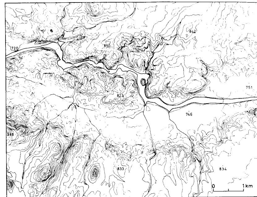
Fig. 12 — Pormenor do graben do Ruacanã. Notar a epigenia e o declive das escarpas. Curvas de nível equidistantes de 10 m.
