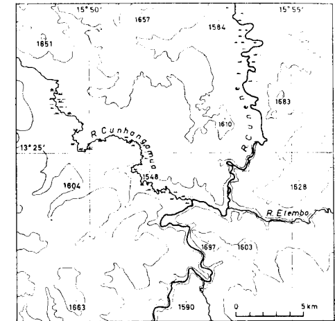
Fig. 5 — Curso superior do Cunene: traçado com faixas de alagadiços e inúmeras curvas.
