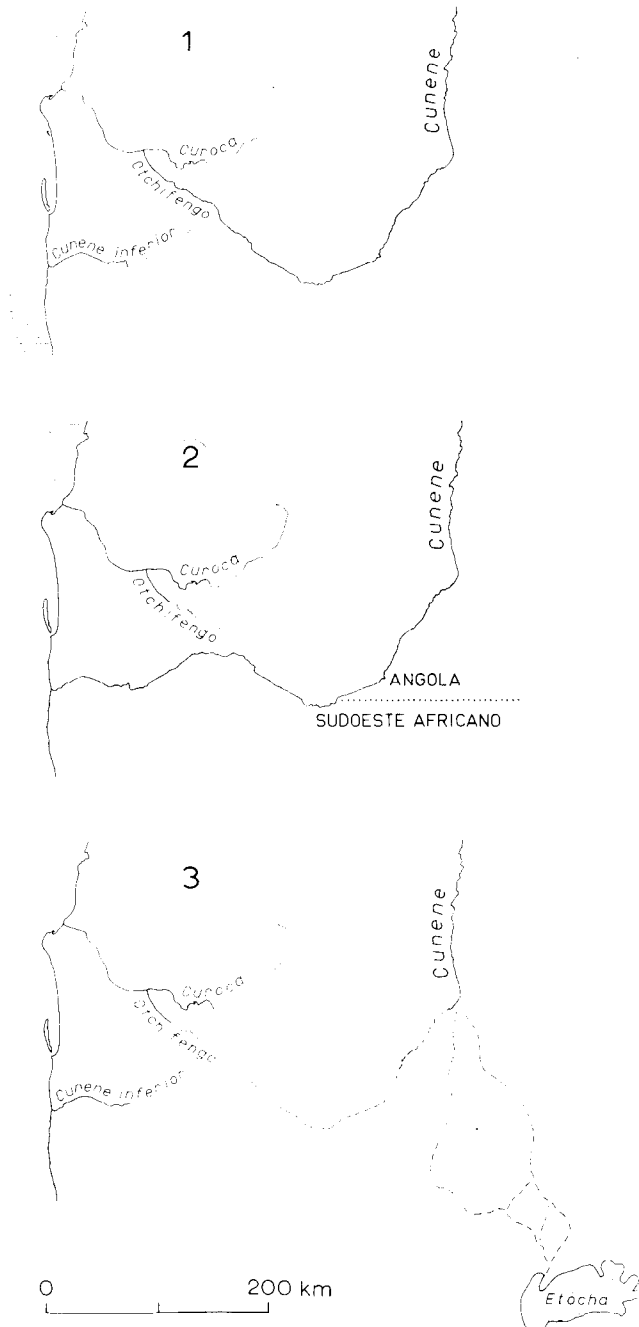
Fig. 15 — A captura do Cunene. 1 — Antigo curso do rio, de acordo com a opinião de BEETZ: o Cunene dirigia-se para o Curoca; 2 — cursos actuais destes rios; 3 — curso antigo do Cunene, segundo a maneira de ver que se defende no presente trabalho.
