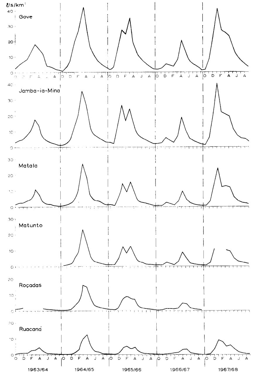
Fig. 3 — Caudais unitários do Cunene (em litros por segundo e por quilômetro quadrado da bacia).
