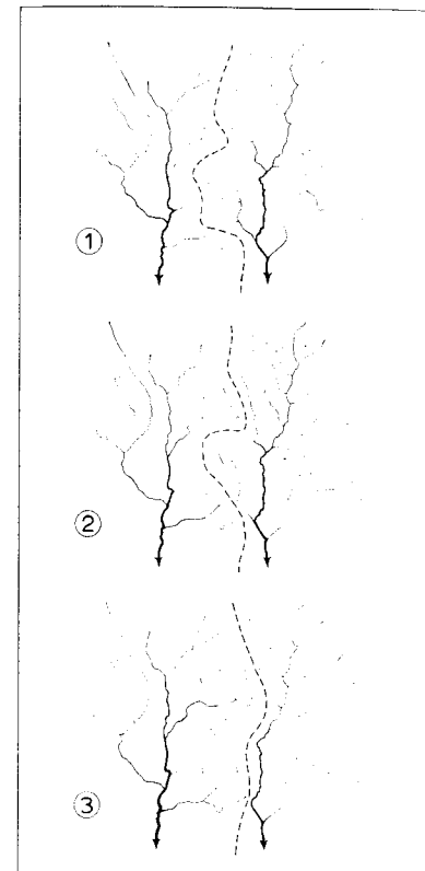
Fig. 16 — Esquema teórico de luta de dois cursos de água pela rede de drenagem.
