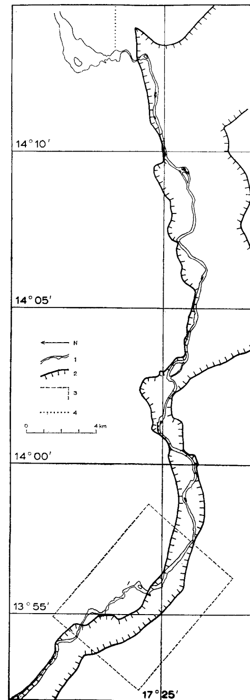
Fig. 10 — O graben do Ruacaná. 1 — Rio; 2 — escarpa; 3 — limites da parte ampliada na fig. 12; 4 — fronteira entre Angola e o Sudoeste Africano.
