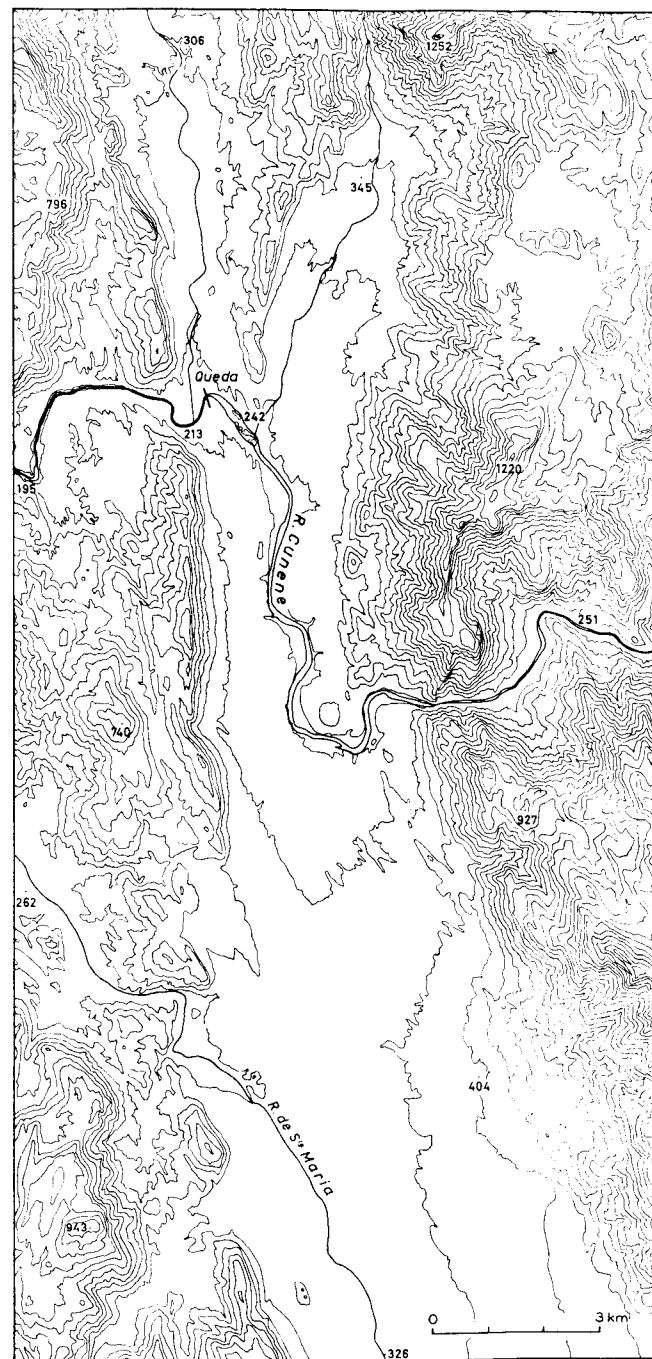
Fig. 13 — O graben do Rio de Santa Maria. Curvas de nível equidistantes de 50 m.
