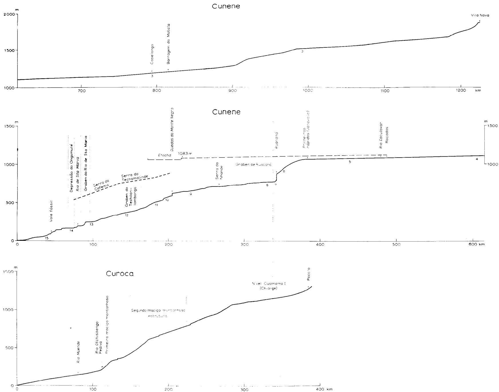
Fig. 6—Perfis longitudinais dos rios Cunene e Curoca.
