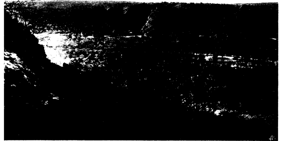
EST. II, A — A extremidade oriental do graben de Ruacanã. Observa-se o fundo do graben , constituído por sedimentos, e a escarpa de falha, de rochas antigas, de um e do outro lado do estreito entalhe (assinalado na fotografia pela seta) por onde o rio entra no graben .
