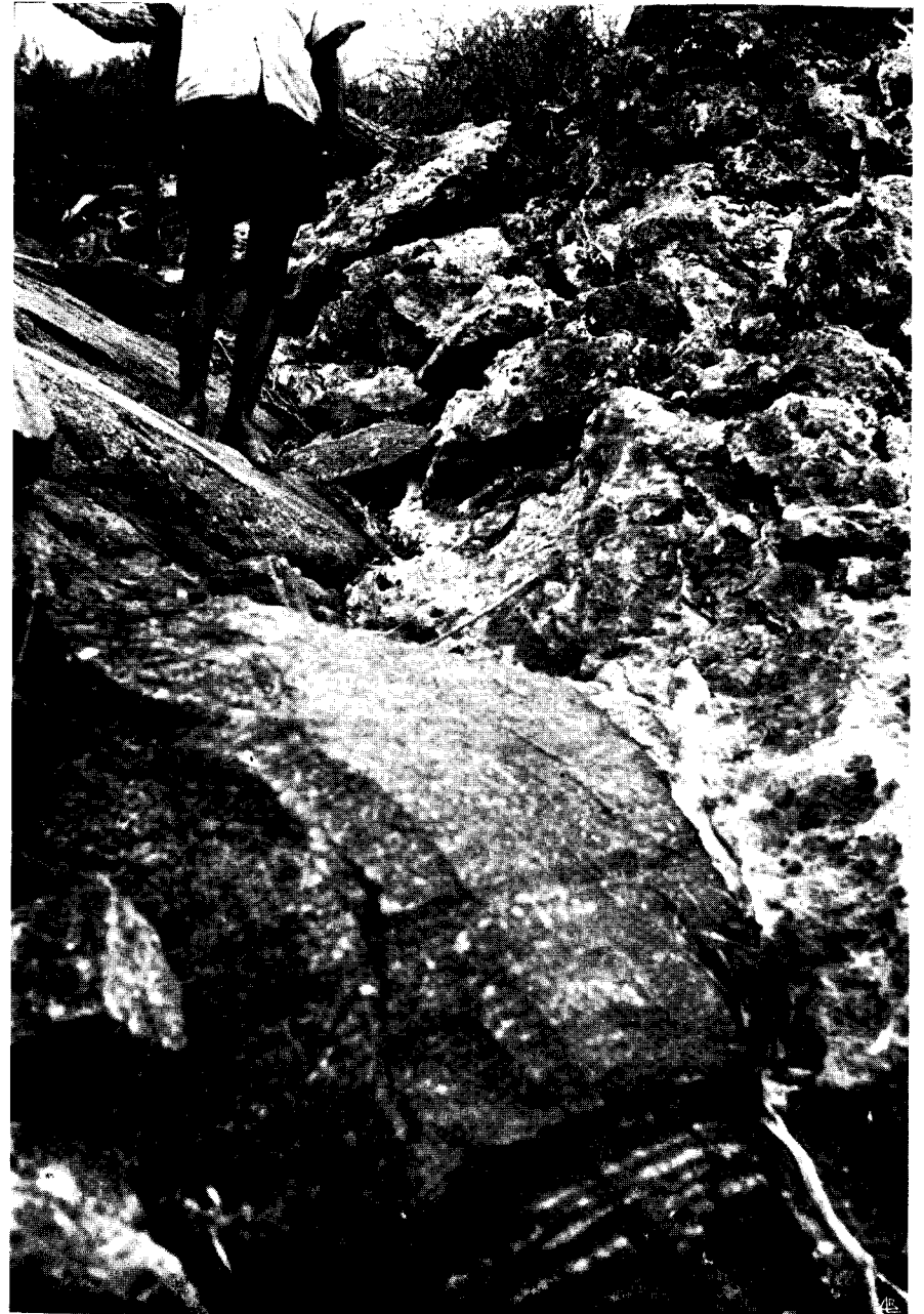
EST. III — A falha do bordo meridional do graben . À direita, os calços sedimentares; à esquerda, as rochas antigas. Observar a estratificação destas e o espelho de falha, especialmente debaixo dos pés do rapaz.
