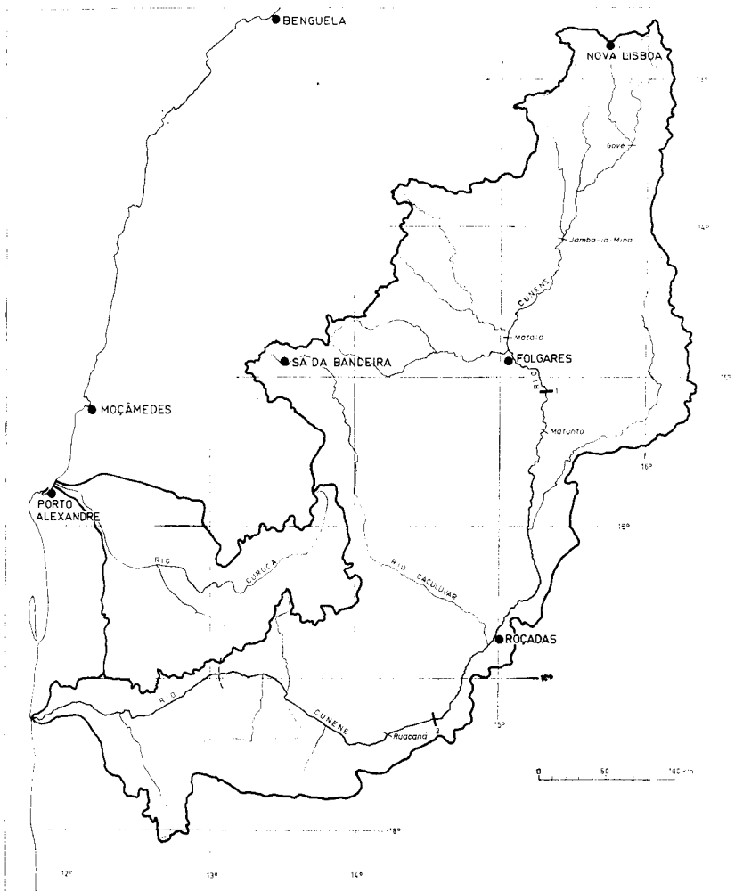
Fig. 1—As bacias hidrográficas dos rios Cunene e Curoca. Os traços assinalados com os números 1 (a jusante de Folgares) e 2 (a jusante de Roçadas) indicam os limites dos cursos superior, médio e inferior do primeiro rio. A linha tracejada, situada a 13° E, marca o limite ocidental da sedimentação endorreica do Cuanhama na maior extensão.
