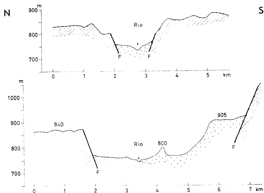
Fig. 11 — Cortes geológicos esquemáticos através do graben do Ruacanã.
