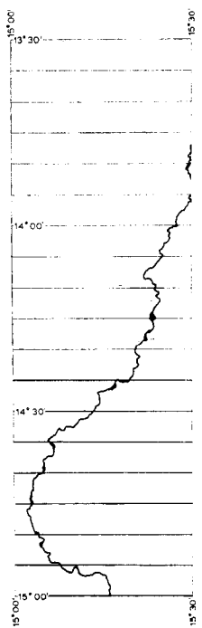
Fig. 8 — Faixa com a largura de 30' de longitude dividida em rectângulos de 5' de latitude, utilizada para determinar o declive da aplanção pelo método da estatística de cotas.
