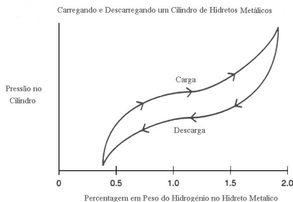
Figura 4 – Variação da pressão e da percentagem em peso do hidrogénio durante a carga e descarga dum cilindro de hidretos metálicos
