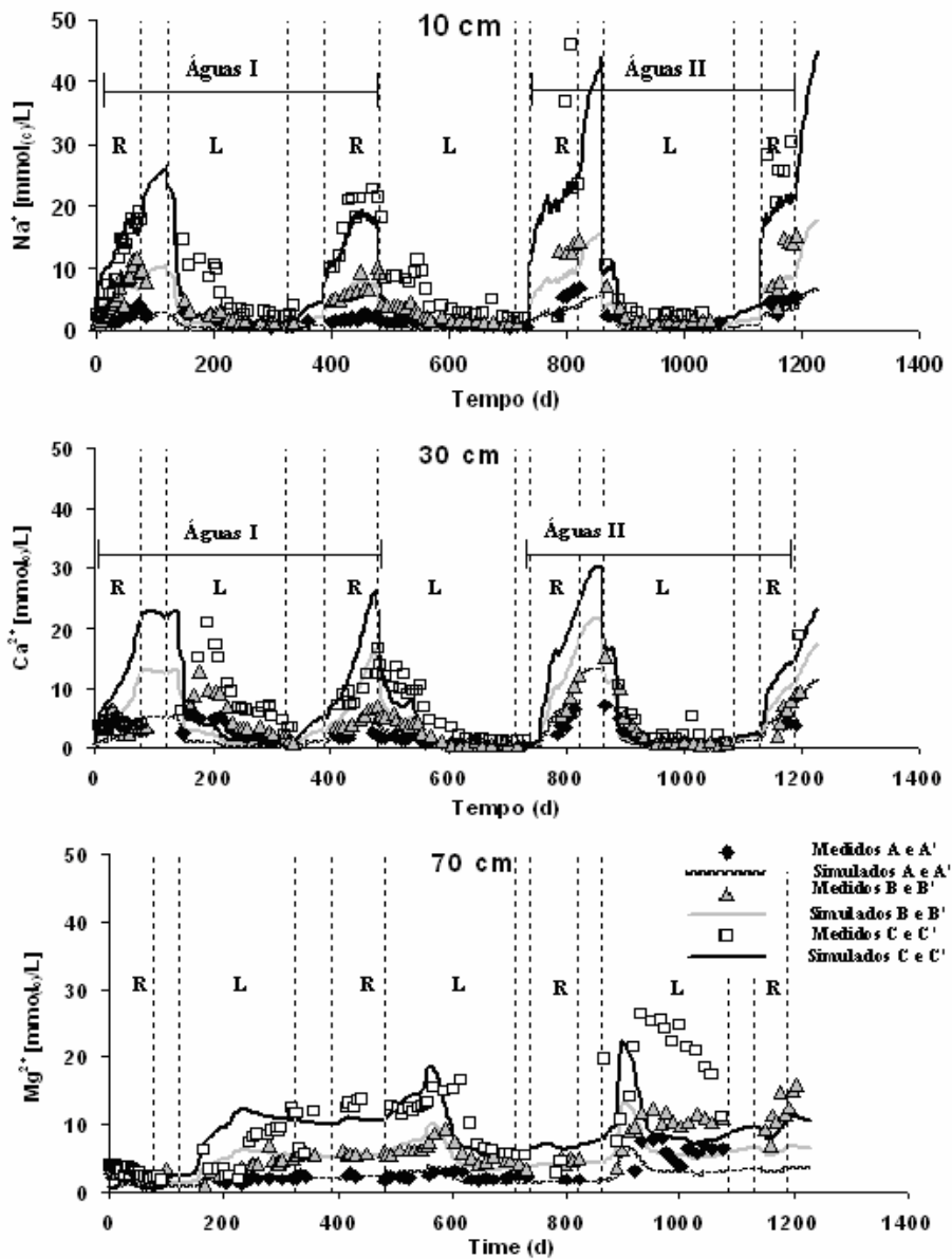
Figura 3 - Exemplos dos resultados da modelação para os teores de sódio, cálcio e magnésio solúveis, nos três monólitos. R corresponde ao período de rega e L ao de lavagem. O período intermédio corresponde aos períodos sem rega nem chuva
