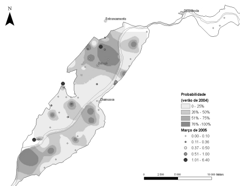
Figura 10 – Variação espacial dos resultados obtidos, relativos aos níveis totais de pesticidas (somatório da concentração dos vários pesticidas detectados, mg/L), na campanha de Março de 2005, sobrepostos à carta de iso-probabilidades calculada para a campanha de 2004 (probabilidade dos níveis totais de pesticidas excederem 0,5mg/L).
