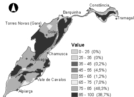
Figura 5 – Mapa que representa a distribuição espacial das classes de susceptibilidade calculadas pelo método IS no sistema aluvionar do Tejo (Adaptado Paralta et al. , 2001).
