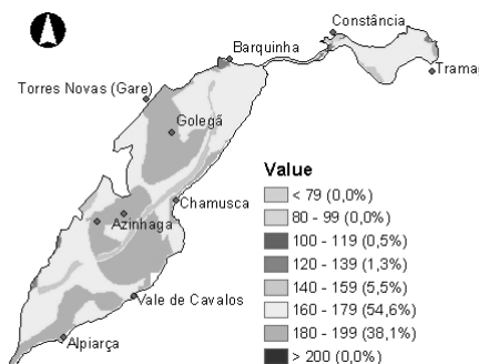
figura 4 – mapa que representa a distribuição espacial das classes de vulnerabilidade obtidas pelo método DRASTIC no sistema aluvionar do Tejo (Adaptado Paralta et al. , 2001).
