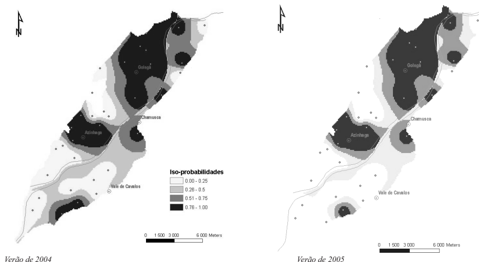
Figura 9 – Mapas de iso-probabilidades das concentrações de nitratos excederem os 50 mg/l na ZVT.
