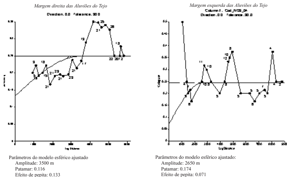
Figura 8 – Semi-variogramas experimentais omnidireccionais e respectivos modelos ajustados para a variável indicatriz de nitrato (Verão 2004).
