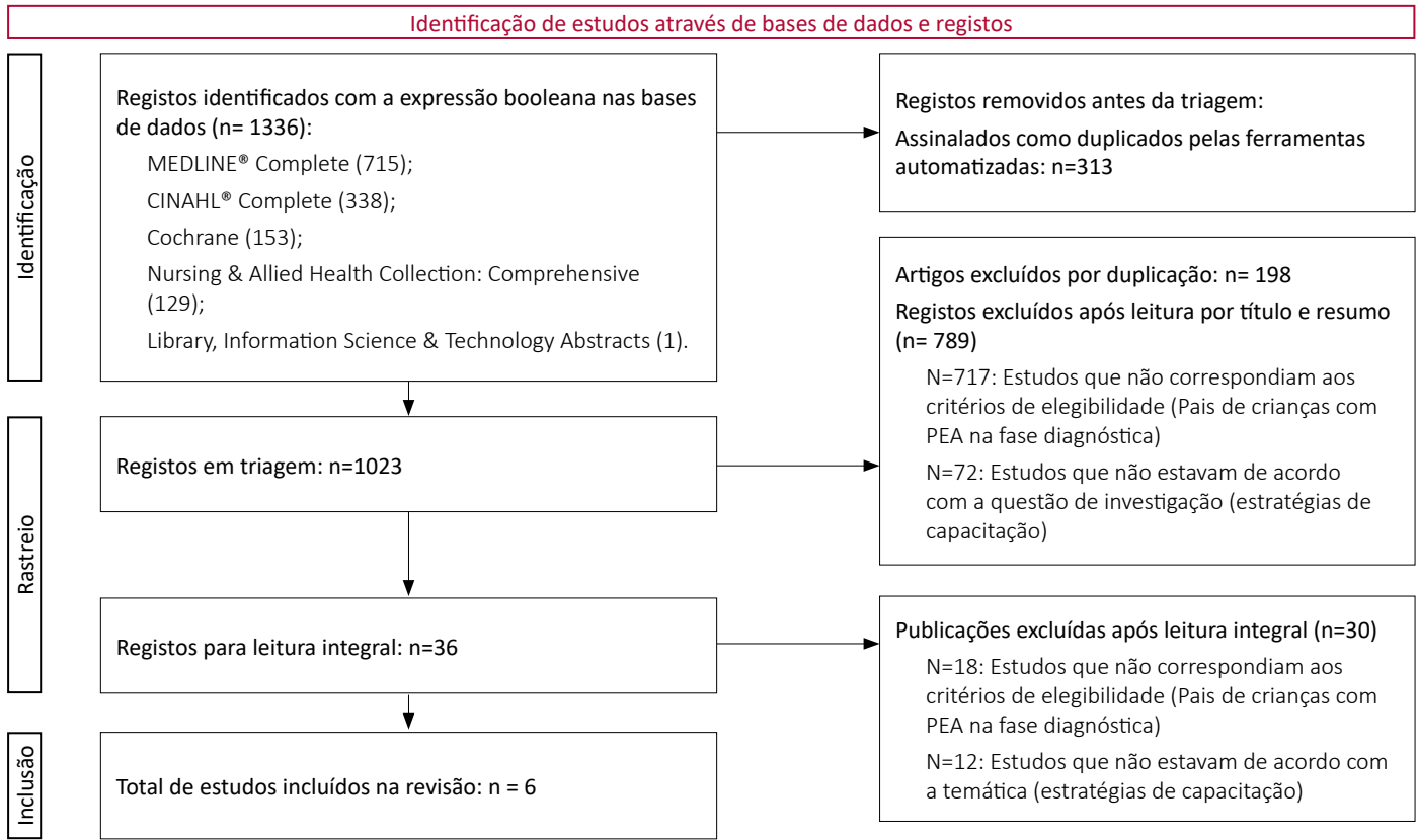
Figura 1- Fluxograma PRISMA-ScR®
